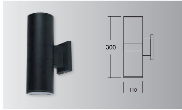
CT-61602 光源：E27*2(另計) 電壓：100V~220V 燈體材質：壓鑄鋁(砂黑烤漆) 防護等級：IP65
