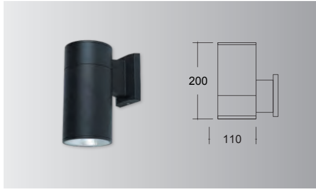
CT-61601 光源：E27*1(另計) 電壓：100V~220V 燈體材質：壓鑄鋁(砂黑烤漆) 防護等級：IP65
