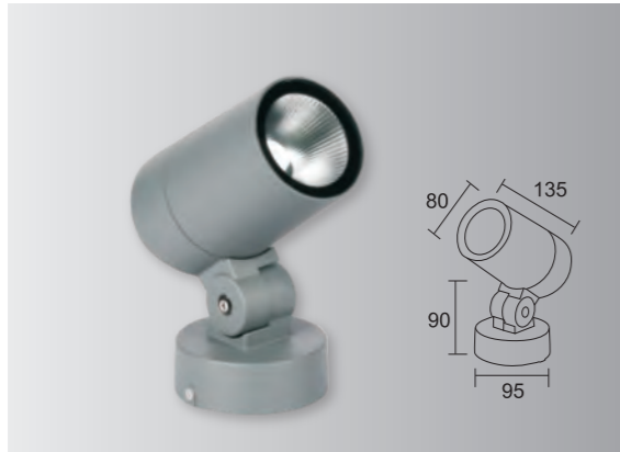
CT-61603 瓦數：12W 材質：鋁製品 色溫：3000K/4000K/5700K 角度：25° /60° 電壓：12V/24V/110V~220V 防護等級：IP65
